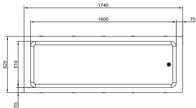
Boven aanzicht
